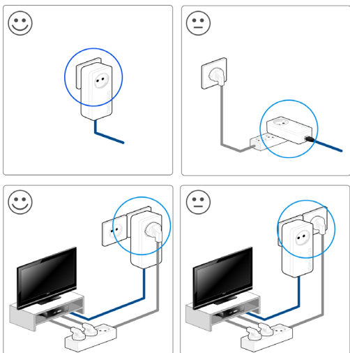
Afb. 5 Optimalisering bandbreedte
